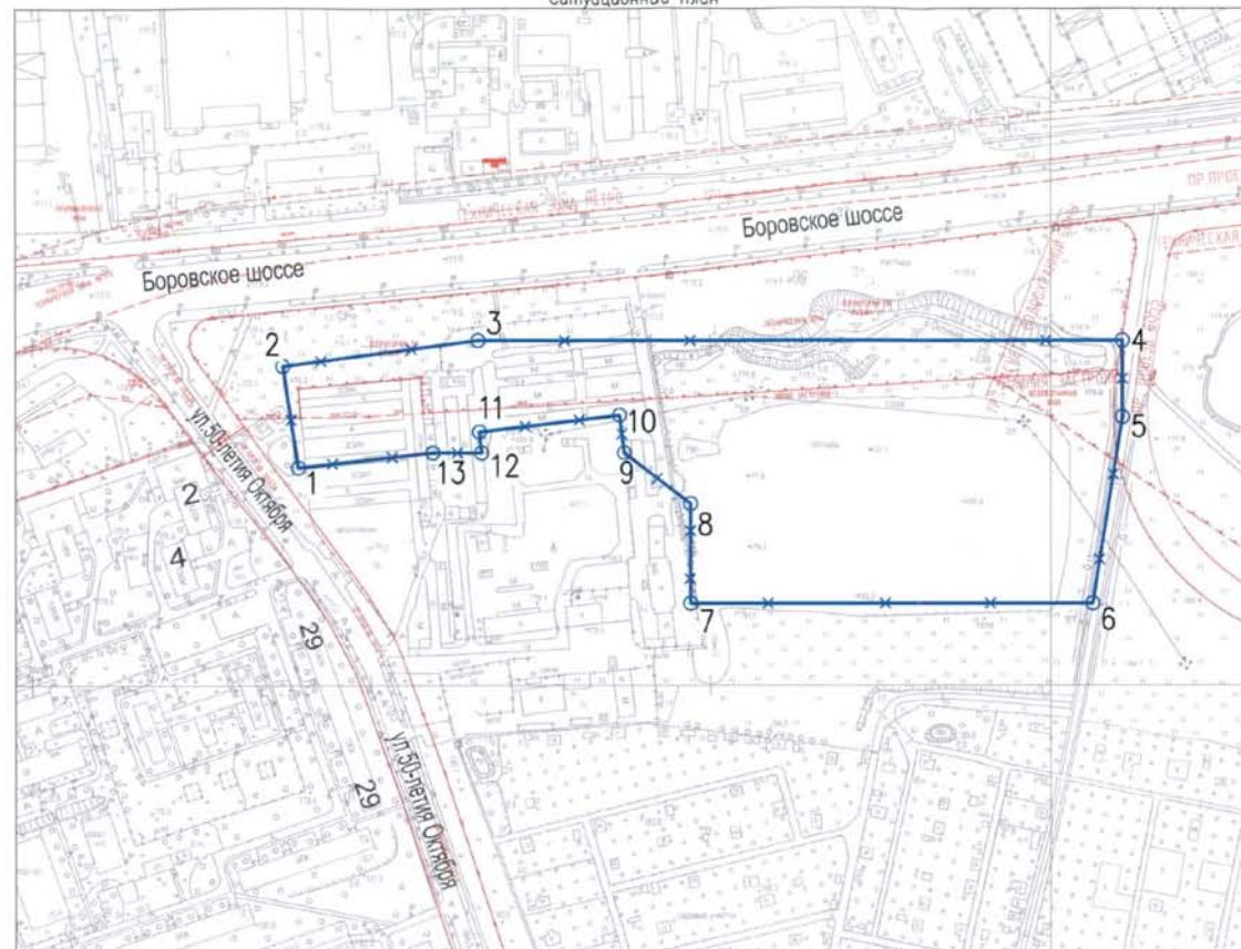
Ситуационный план
